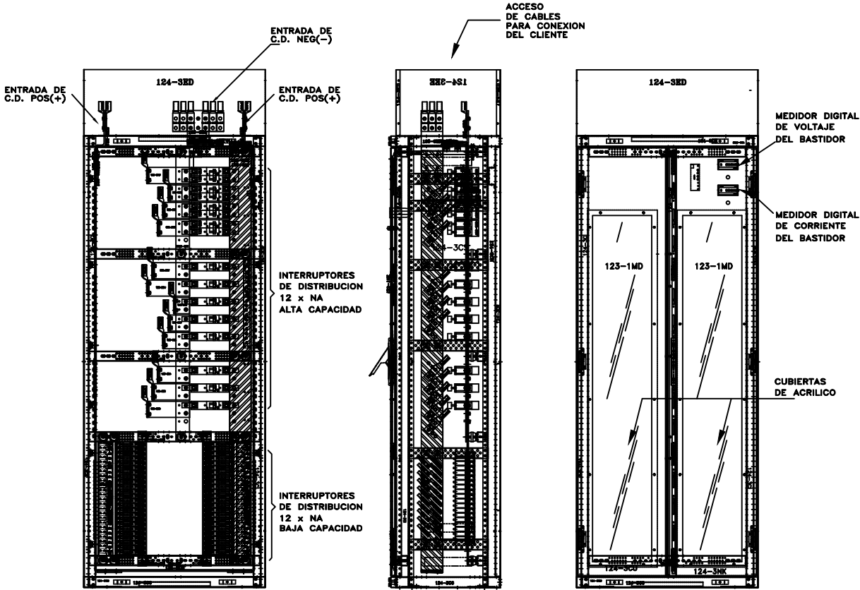
VISTA FRONTAL ( SIN PUERTAS )
